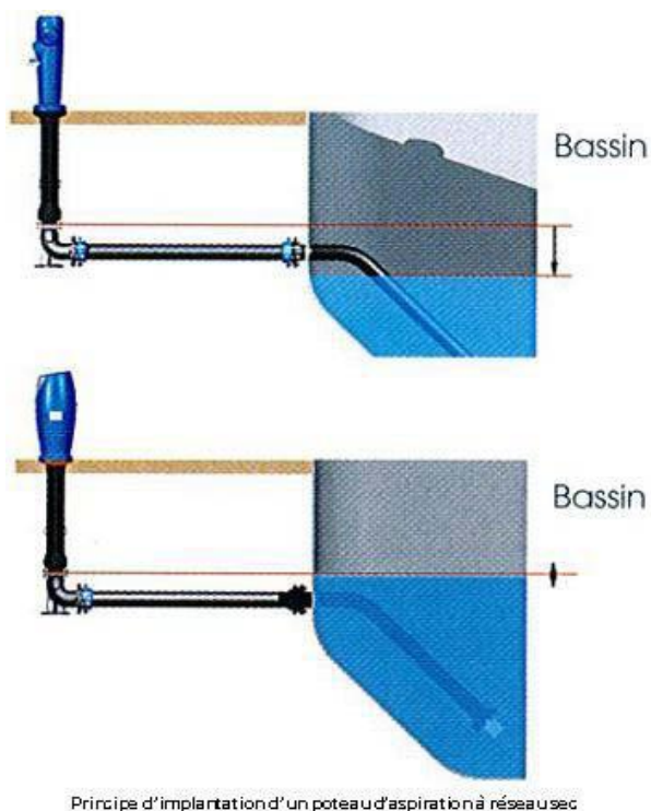
Principe d'implantation d'un poteau d'aspiration à réseau sec
